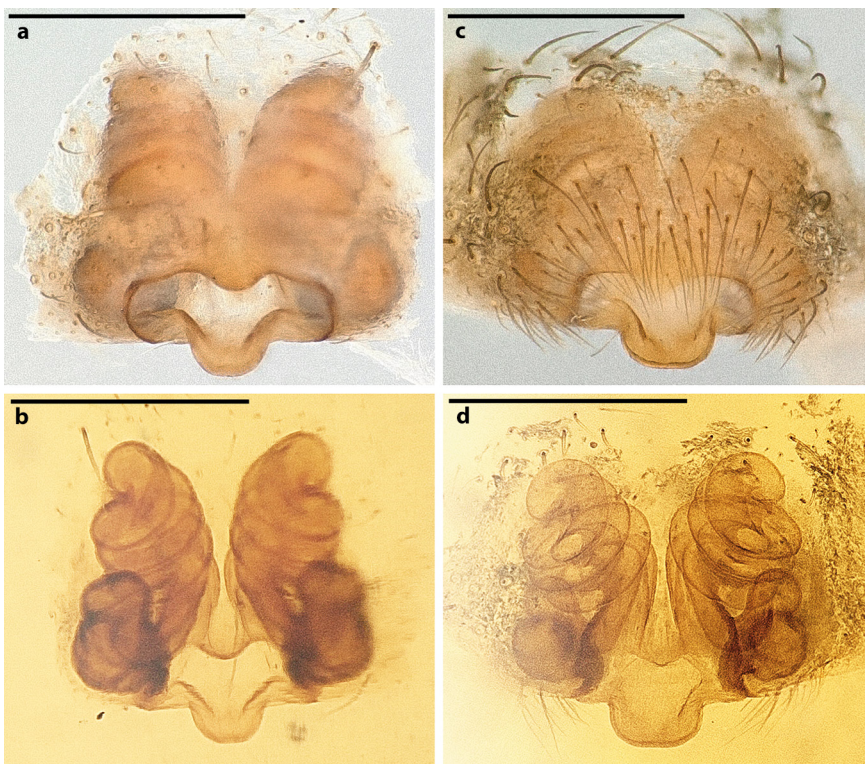
Abb. 2: Epigyne und Vulva; a, c. Ventral; b, d. Dorsale Sicht, mit Nelkenöl aufgehellt; a-b. Tetrax caudata , Italien; c-d. Tetrax cf. rubrofoliata , Spanien. Indikator-Balken entspricht 0.5 mm
