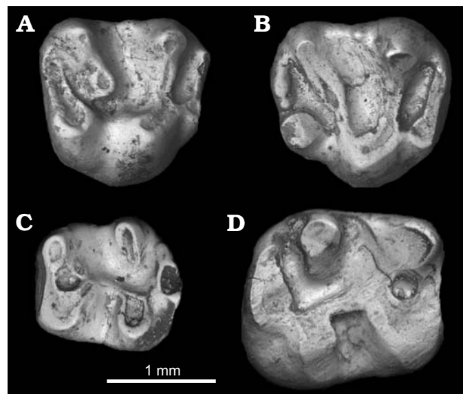
Fig. 13. Ctenodactyloid rodent Gobiomys exiguus Wang, 2001 from the Eocene of Wulanhuxiu, Nei Mongol, China. A. Right M2 (IVPP V20827.1). B. Right M3 (IVPP V20827.2). C. Left m1 (IVPP V20827.3). D. Right m2 (IVPP V20827.4). All in occlusal view.
