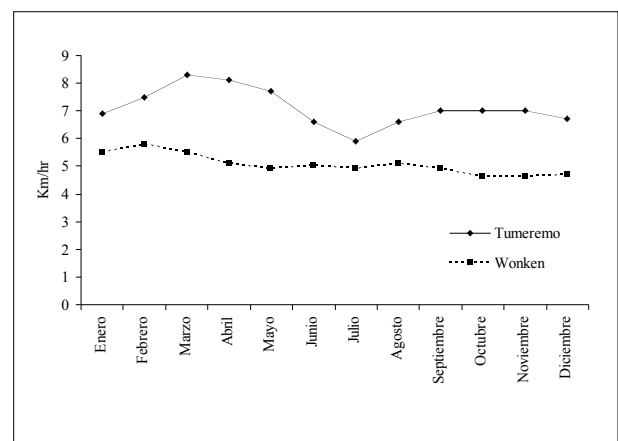
Figura 1.8. Velocidad del viento promedio mensual en las estaciones metereológicas de Tumeremo (07° 18' N- 61° 073' W-180 m s.n.m.) y Wonkén (844 m s.n.m.- coordenadas no disponibles), para los periodos (1951-1990 y 1982-1999, respectivamente). Fuente: (CABC-IC 2005).
