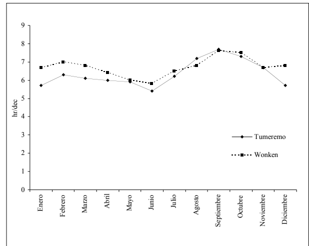
Figura 1.6. Insolación promedio mensual en las estaciones metereológicas de Tumeremo (07° 18' N- 61° 073' W-180 m s.n.m.) y Wonkén (844 m s.n.m.- coordenadas no disponibles), para los periodos (1995-1999 y 1982-2000, respectivamente). Fuente: (CABC-IC 2005).
