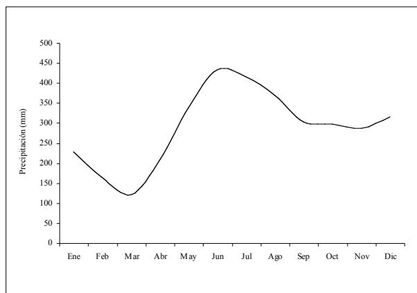
Figura 1.1. Precipitación promedio mensual (1994-2008) en la Estación Meteorológica Las Brisas ( 06^{\circ} 10' 02'' N – 61^{\circ} 28' 18'' W). Fuente: (CABC-IC 2005).
