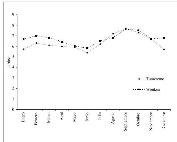
Figura 1.6. Insolación promedio mensual en las estaciones metereológicas de Tumeremo (07° 18' N- 61° 073' W-180 m s.n.m.) y Wonkén (844 m s.n.m.- coordenadas no disponibles), para los periodos (1995-1999 y 1982-2000, respectivamente). Fuente: (CABC-IC 2005).
