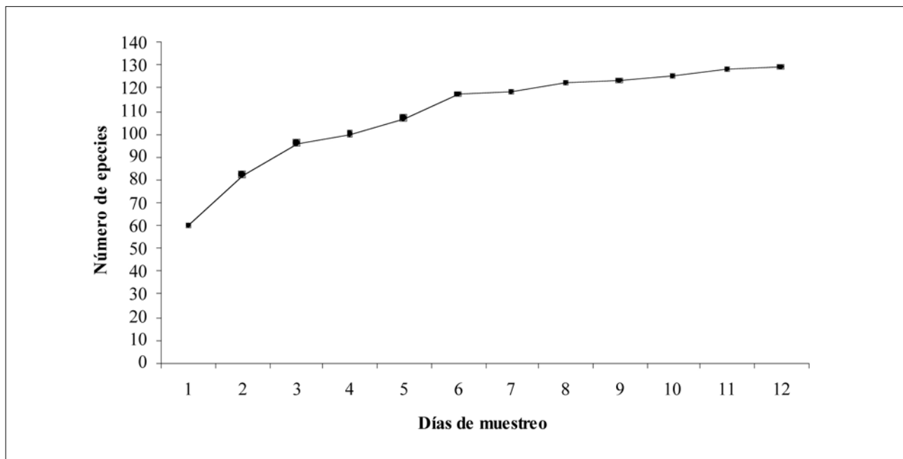
Figura 6.1. Curva acumulada de especies de peces en función de los días de muestreo del RAP Alto Cuyuní 2008.
