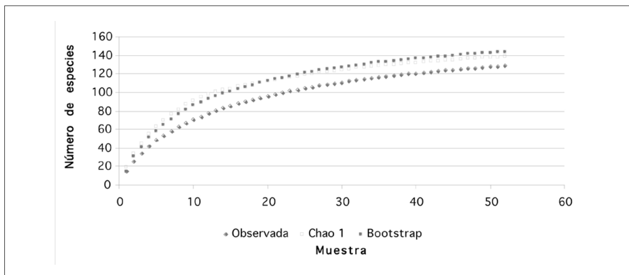
Figura 6.2. Curva de acumulación de especies probables para las cuencas del río Cuyuní-Uey (RAP Alto Cuyuní 2008).
