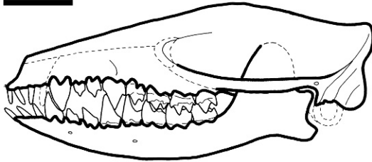
Kennalestes gobiensis
