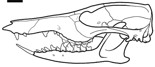
Zalambdalestes lechei
