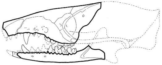
Zalambdalestes lechei
