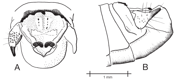
Fig. 11. Cryptacris costaricensis . Male terminalia. A. Dorsal view B. Lateral view.
