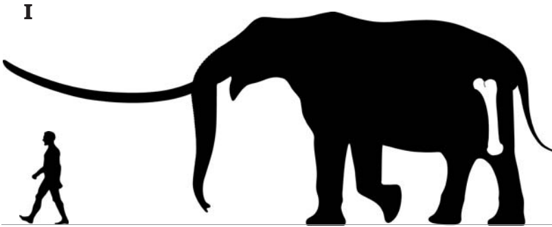
SH ~410 cm • BM ~16 t
