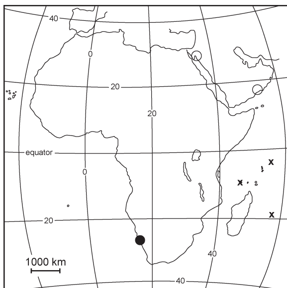
Fig. 70. Distribution of Krifomyia gen. n. (●), Paraphanosoma gen. n. (x), and Tethysimyia gen. n. (○).
