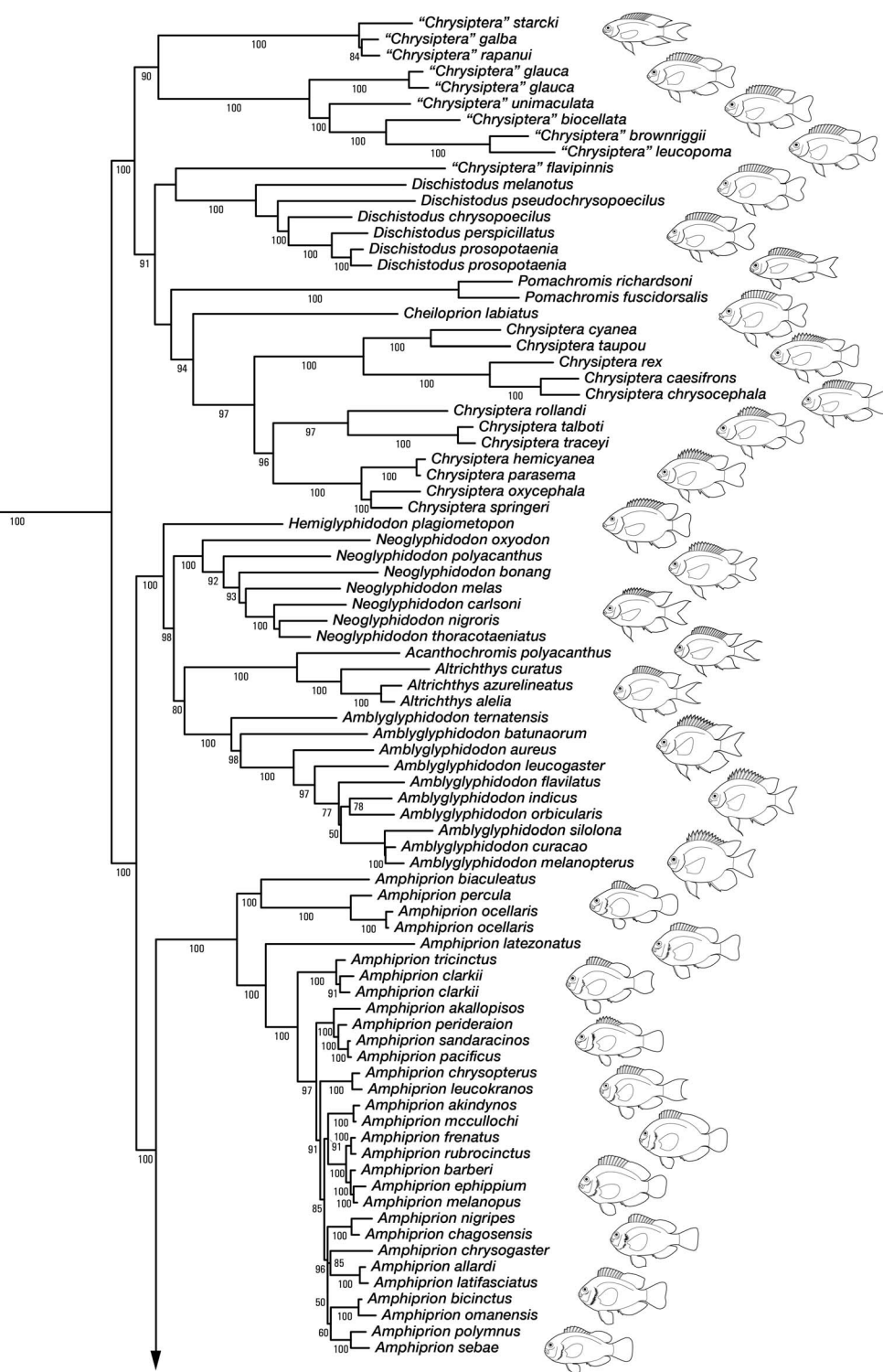
D POMACENTRINAE (continued) Fig. 1. (continued). N. nigroris , Acanthochromis polyacanthus , Altrichthys azurelineatus , Amblyglyphidodon aureus , A. curacao , A. orbicularis , Amphiprion ocellaris , A. latezonatus , A. clarkii , A. perideraion , A. chrysopterus , A. frenatus , A. ephippium , A. chrysogaster , A. bicinctus , A. polymnus ; (E) Amblypomacentrus tricinctus , A. breviceps , Pristotis obtusirostris , Teixeirichthys jordani , Neopomacentrus bankieri , N. filamentosus , N. xanthurus , N. miryae , N. metallicus , N. azysron , Pomacentrus pavo , P. caeruleus , P. auriventris , P. coelestis , P. aquilus , P. trilineatus , P. chrysurus , P. vaiuli , P. bankanensis , P. amboinensis , P. moluccensis , P. tripunctatus , P. taeniometopon , P. callainus , P. brachialis , P. nagasakiensis , P. stigma , P. nigromanus , P. philippinus , P. imitator . See Data Accessibility for tree file.
