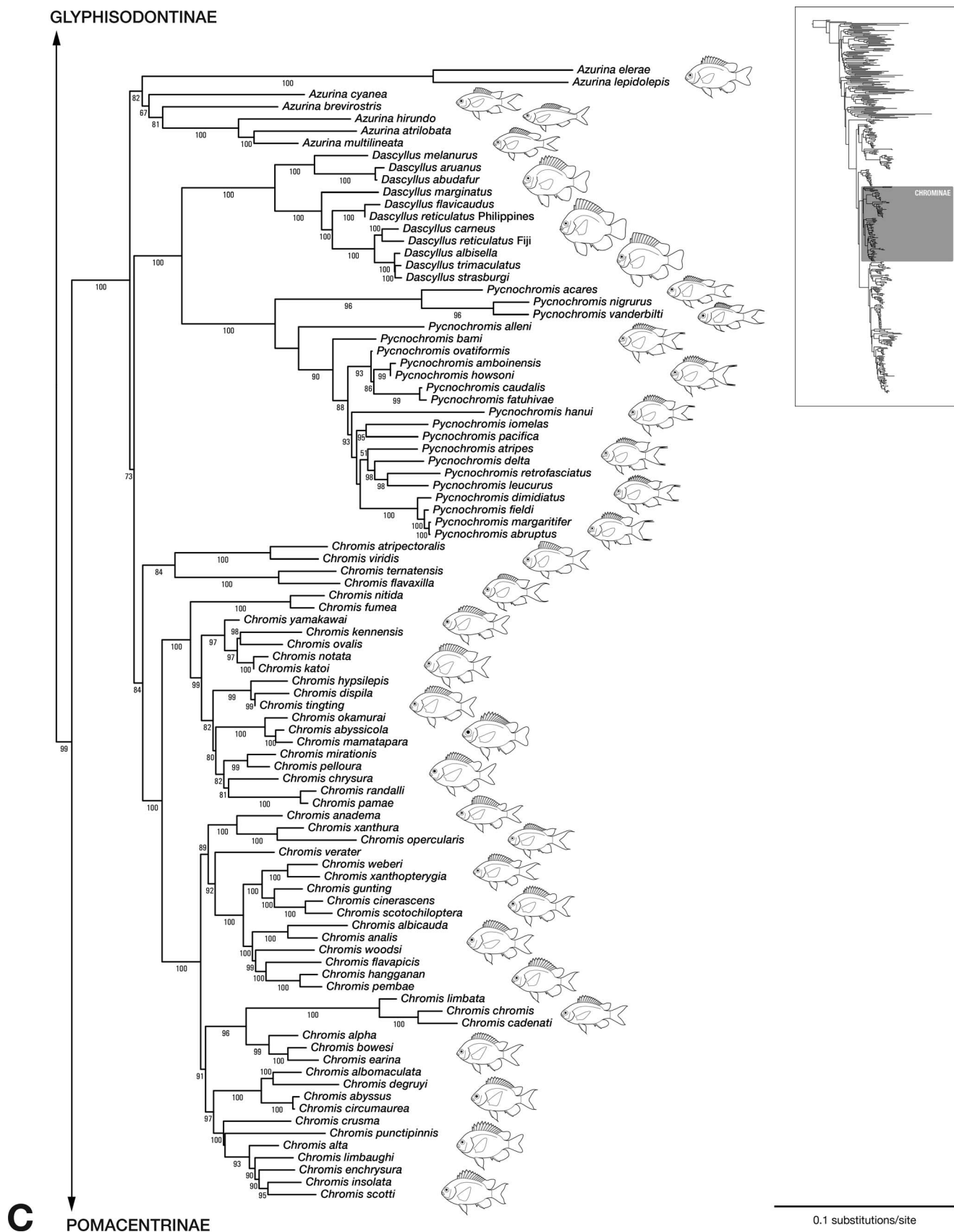
Fig. 1. (continued). P. hanui , P. atripes , P. fieldi , P. margaritifera , Chromis viridis , C. ternatensis , C. fumea , C. notata , C. hypsilepis , C. okamurai , C. chrysura , C. randalli , C. opercularis , C. weberi , C. cinerascens , C. analis , C. pembae , C. chromis , C. alpha , C. abyssus , C. alta , C. insolata ; (D) " Chrysiptera " rapanui , " C. " glauca , " C. " biocellata , " C. " brownriggii , Dischistodus chrysopoecilus , D. prosopotaenia , Pomachromis richardsoni , Cheiloprius labiatus , Chrysiptera cyanea , C. rex , C. traceyi , C. oxycephala , Hemiglyphidodon plagiometopon , Neoglyphidodon polyacanthus ,
