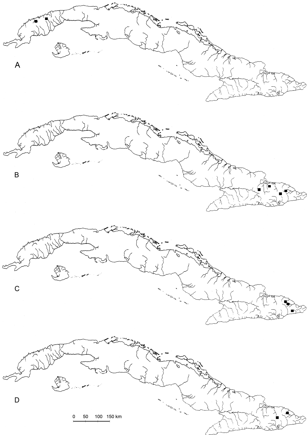
Fig. 11. Distribution of the species of Tylodontia – A: T. cubensis ; B: T. fuscata ; C: T. stipitata ; D: T. urceolata .
